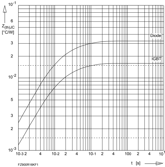
Bild/Fig. 5 Transient inner thermal impedance (DC) Transient thermal impedance (DC)
