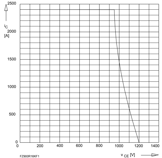
Bild/Fig. 4 Rückwärts-Arbeitsbereich Reverse biased safe operating area t_{vj} = 125\text{ °C} , v_{LF} = v_{LR} = 15V , R_G = 0,82\text{ }\mu
